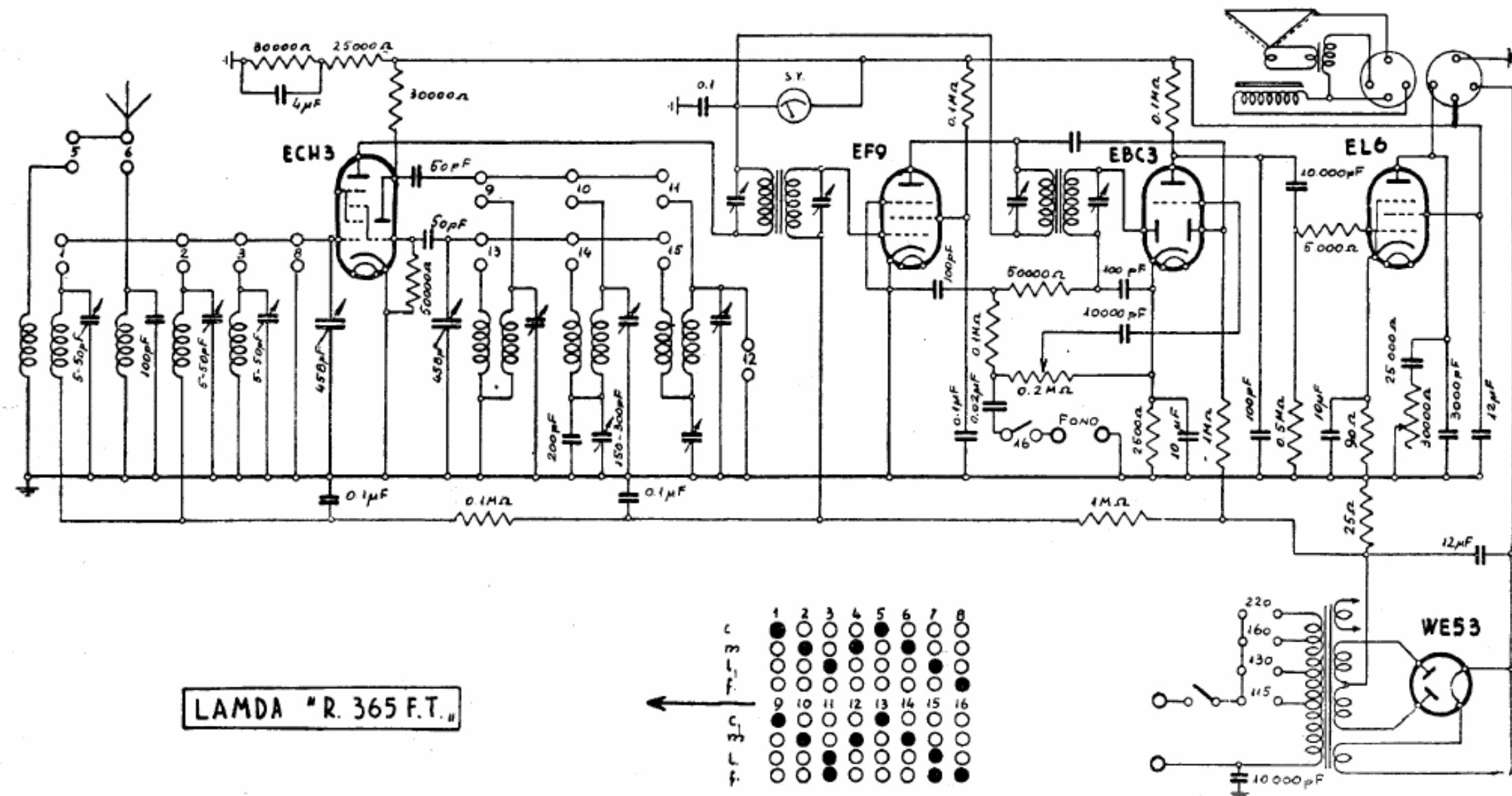
LAMBDA (Olivieri e Glisenti). — Mod. « Lambda 365 F.T. ». — Produzione 1939-1940. — Media frequenza: 465 kHz.
